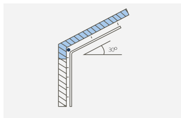
INCLINADO
