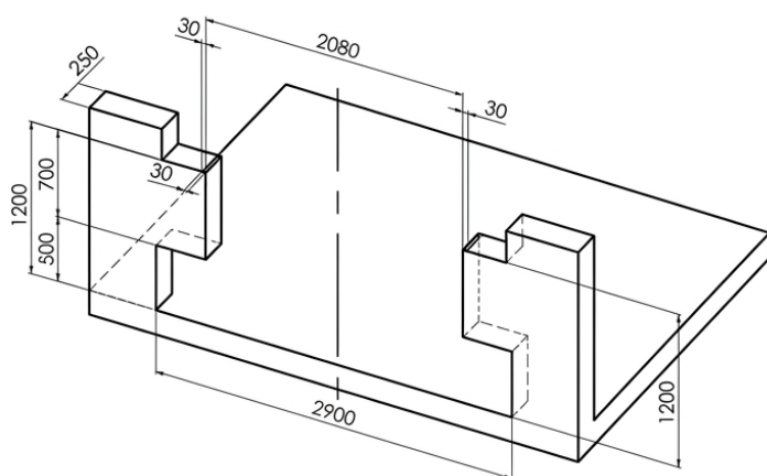
DIMENSIONES PARA CAJÓN ENCOFRADO
