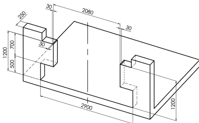
DIMENSIONS DE LA FOSSE COFFRAGE
